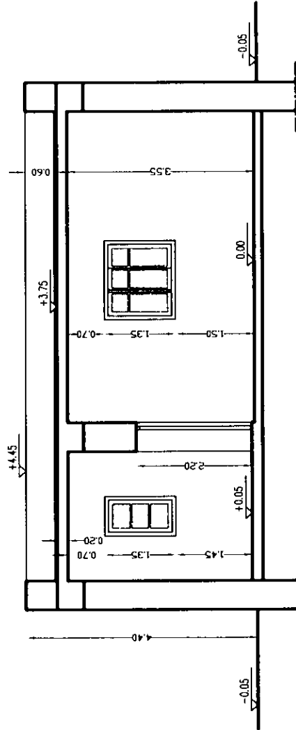
ΤΟΜΗ α-α'
